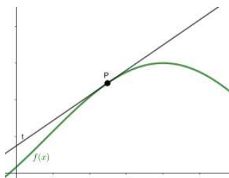
Funció còncava
