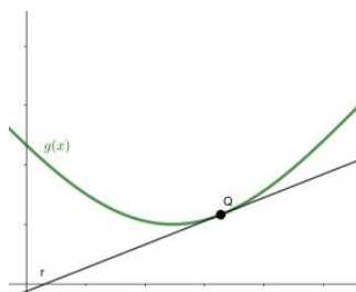
Funció convexa
