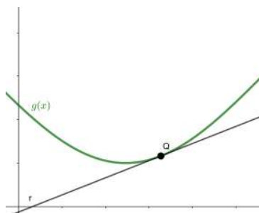
Funció convexa
