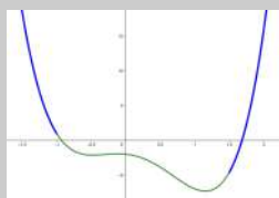
f(x)
