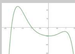
h(x)
